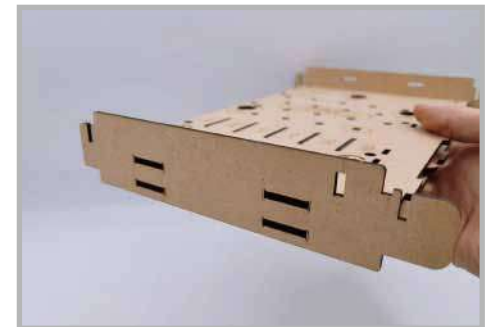
15 將零件26安裝至對應的位置·注意組裝方向
