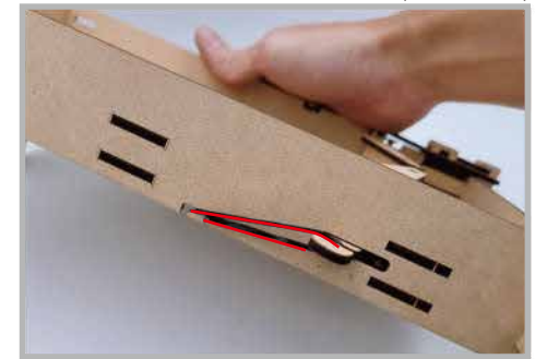
30 另一側的橡皮筋也套至對應的位置(紅線標示處)
