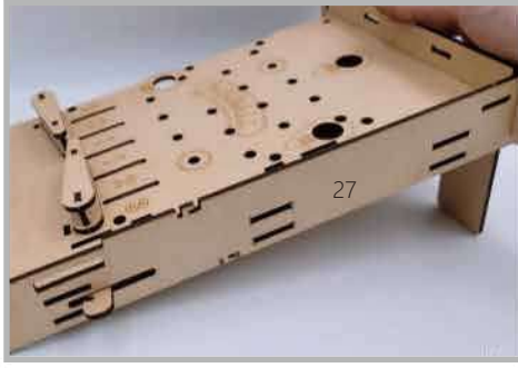
17 零件27安裝至對應的位置
