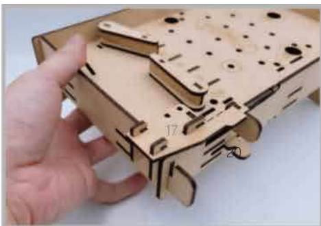
25 零件17安裝至對應位置
