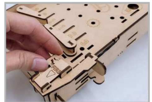
27 零件19安裝至零件17上對應的孔洞，將零件31固定
