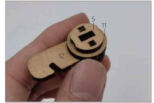
9 零件12、零件11、零件5安裝至對應的孔洞
