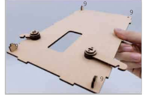
12 將零件9、及完成的手把安裝至零件2對應的孔洞
