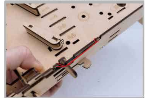
24 沿著圖片標示套上橡皮筋(紅線處)
