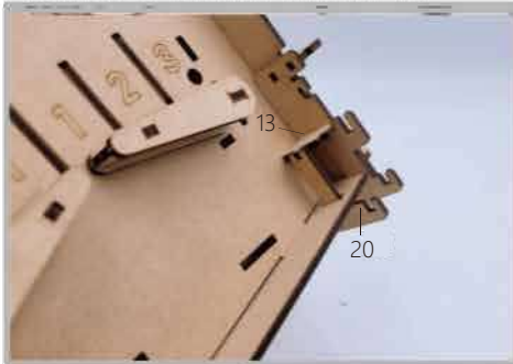
23 零件13安裝在對應的位置，零件20穿過底板孔洞與零件13組合
