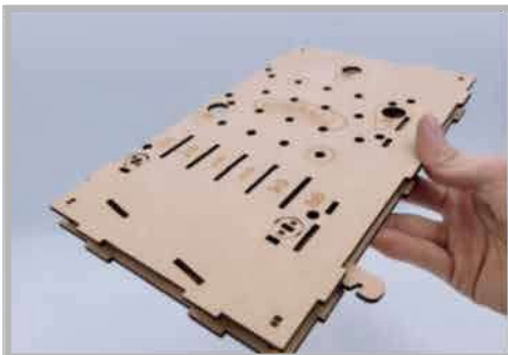
13 零件1與零件2組合在一起
