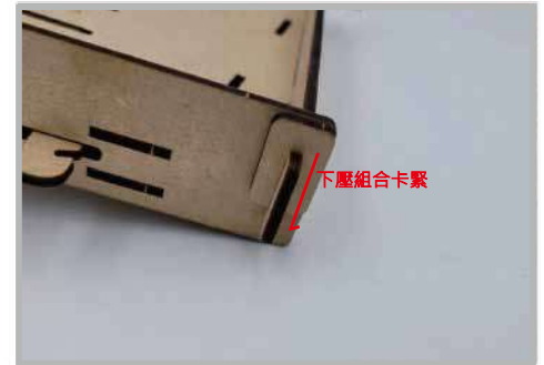
21 零件30安裝至側板對應的孔洞與零件26進行組合
